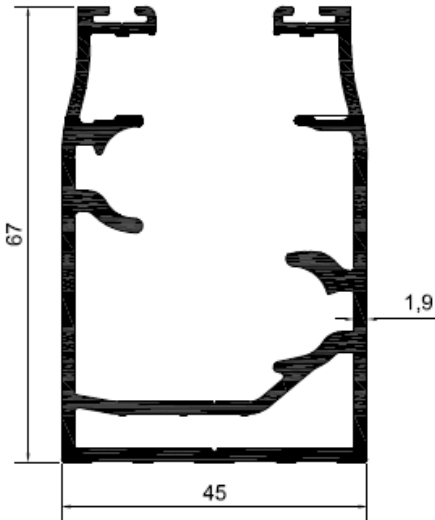
Profil No: N5148 Gramaj : 1,550 kg/mt
