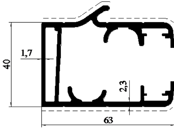
Profil No: 7766 Gramaj : 1,580 kg/mt
