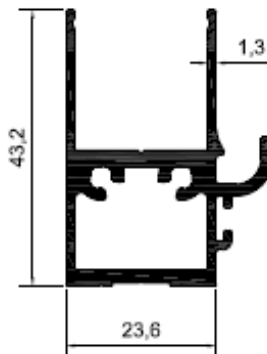
Profil No: N5336 Gramaj : 0,781 kg/mt
