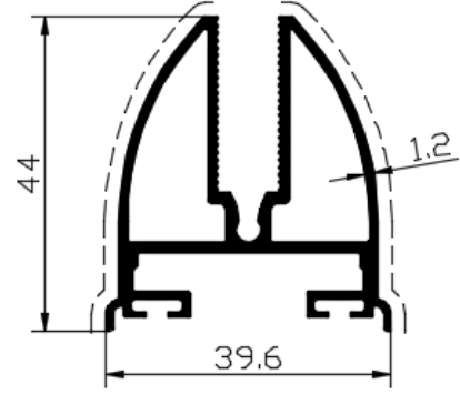
Profil No: 7477 Gramaj : 0,813 kg/mt
