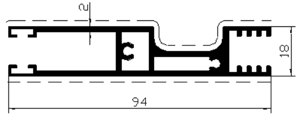
Profil No: 7159 Gramaj : 1,215 kg/mt
