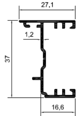
Profil No: N5142 Gramaj : 0,335 kg/mt
