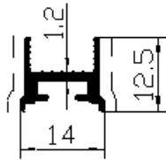
Profil No: 7156 Gramaj : 0,130 kg/mt
