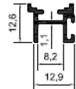
Profil No: N5217 Gramaj : 0,155 kg/mt
