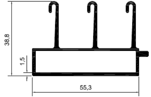
Profil No: N5221 Gramaj : 0,975 kg/mt
