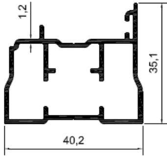
Profil No: N5149 Gramaj : 0,560 kg/mt
