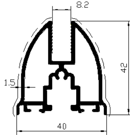
Profil No: 6094 Gramaj : 0,938 kg/mt
