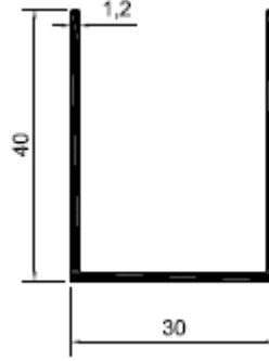
Profil No: N1521 Gramaj : 0,400 kg/mt
