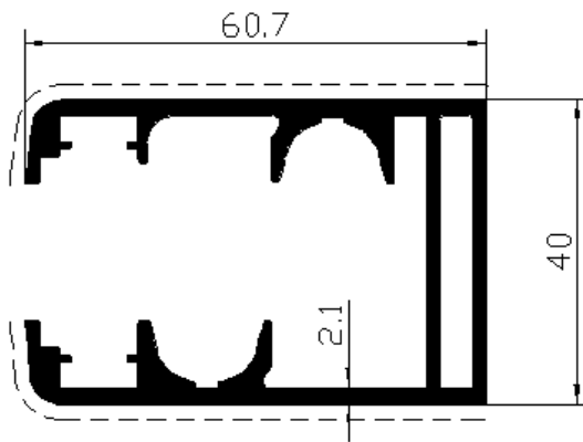
Profil No: 7650 Gramaj : 1,461 kg/mt
