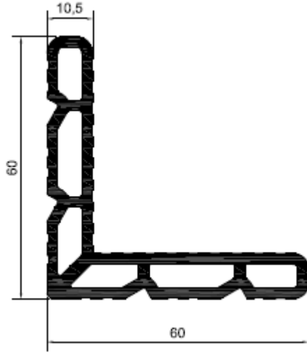
Profil No: N5337 Gramaj : 1,670 kg/mt
