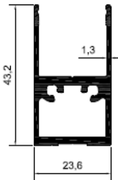
Profil No: N5149 Gramaj : 0,560 kg/mt
