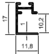
Profil No: N5218 Gramaj : 0,128 kg/mt
