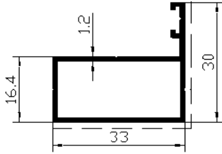
Profil No: 6089 Gramaj : 0,369 kg/mt
