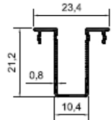
Profil No: N5339 Gramaj : 0,155 kg/mt
