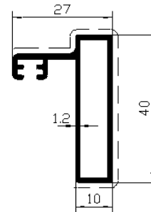
Profil No: 6096 Gramaj : 0,439 kg/mt
