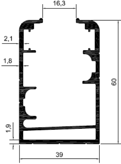
Profil No: 5120 Gramaj : 1,240 kg/mt
