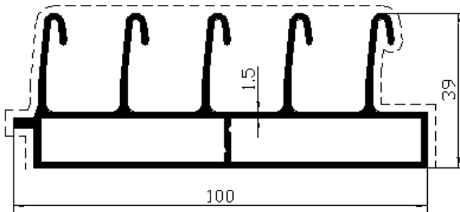
Profil No: 7152 Gramaj : 1,667 kg/mt
