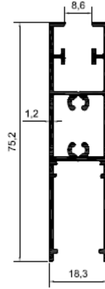
Profil No: N5235 Gramaj : 0,736 kg/mt
