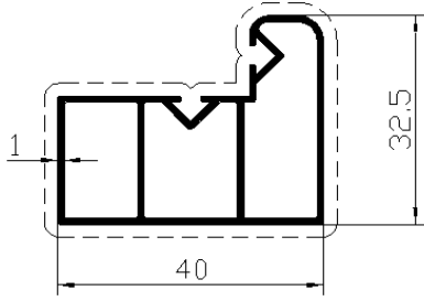
Profil No: 7478 Gramaj : 1,309 kg/mt
