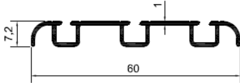
Profil No: N5222 Gramaj : 0,300 kg/mt
