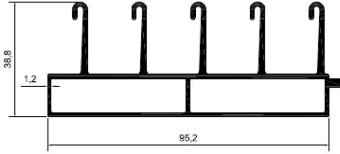
Profil No: N5212 Gramaj : 1,590 kg/mt
