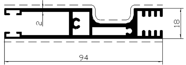
Profil No: 7159 Gramaj : 1,215 kg/mt
