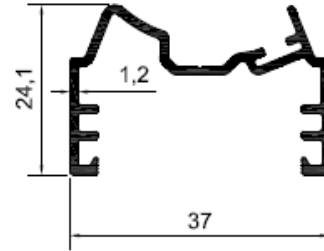
Profil No: N5152 Gramaj : 0,344 kg/mt
