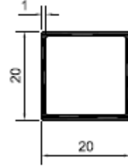
Profil No: N5338 Gramaj : 0,206 kg/mt
