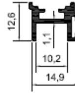
Profil No: N5216 Gramaj : 0,170 kg/mt
