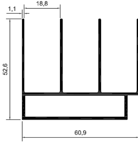
Profil No: N5212 Gramaj : 1,590 kg/mt
