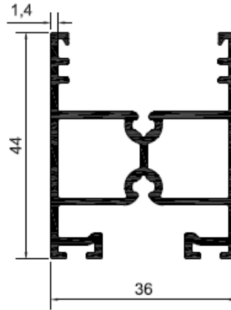
Profil No: N5146 Gramaj : 0,855 kg/mt
