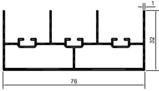
Profil No: N5231 Gramaj : 0,795 kg/mt
