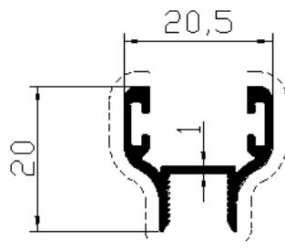
Profil No: 7763 Gramaj : 0,225kg/mt
