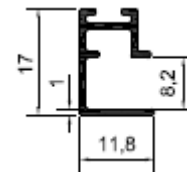
Profil No: N5219 Gramaj : 0,135 kg/mt
