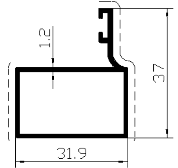
Profil No: 7651 Gramaj : 0,423 kg/mt
