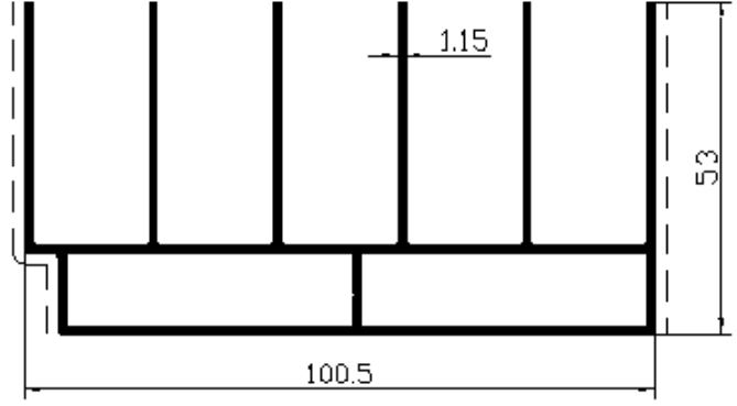
Profil No: 7150 Gramaj : 1,463 kg/mt
