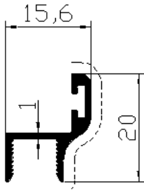
Profil No: 7764 Gramaj : 0,157 kg/mt
