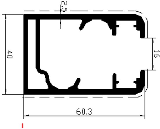
Profil No: 6095 Gramaj : 1,561 kg/mt
