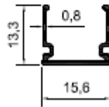
Profil No: N5238 Gramaj : 0,104 kg/mt
