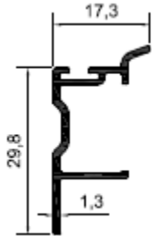
Profil No: N5237 Gramaj : 0,210 kg/mt
