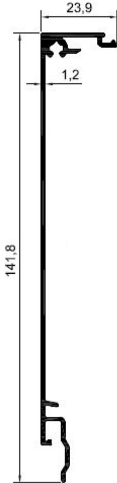
Profil No: N5334 Gramaj : 0,792 kg/mt
