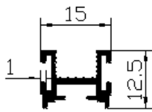
Profil No: 7157 Gramaj : 0,157 kg/mt
