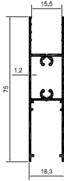
Profil No: N5234 Gramaj : 0,675 kg/mt
