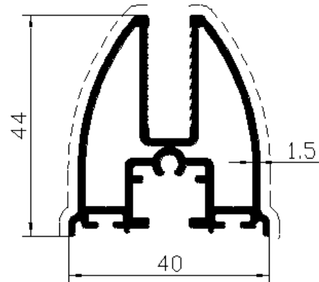
Profil No: 7649 Gramaj : 0,992 kg/mt
