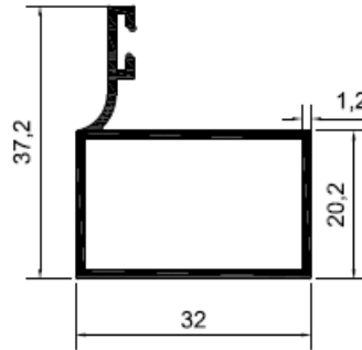
Profil No: 5123 Gramaj : 0,410 kg/mt
