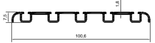
Profil No: N5213 Gramaj : 0,663 kg/mt
