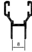
Profil No: N5133 Gramaj : 0,207 kg/mt
