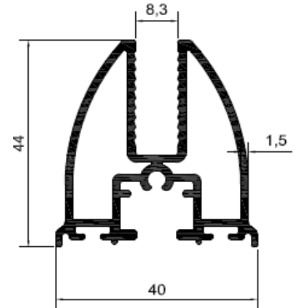
Profil No: 5124 Gramaj : 0,990 kg/mt
