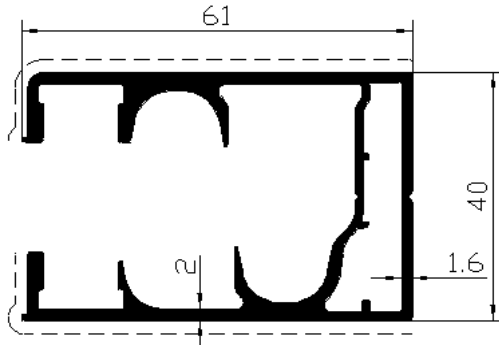
Profil No: 7478 Gramaj : 1,309 kg/mt
