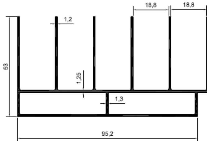
Profil No: N5211 Gramaj : 1,552 kg/mt
