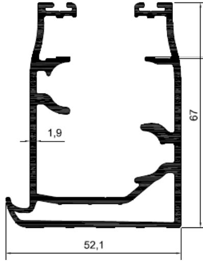
Profil No: N5153 Gramaj : 1,566 kg/mt
