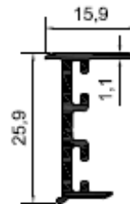
Profil No: N5332 Gramaj : 0,200 kg/mt
