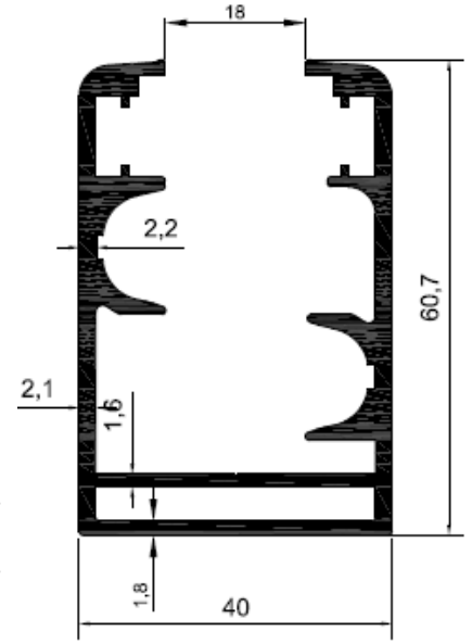
Profil No: 5125 Gramaj : 0,1465 kg/mt
