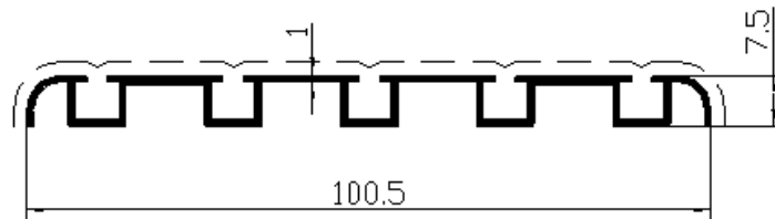
Profil No: 7151 Gramaj : 0,550 kg/mt
