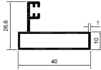
Profil No: 5121 Gramaj : 0,386 kg/mt
