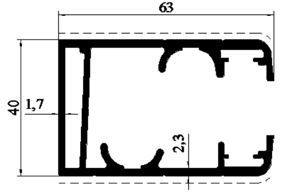
Profil No: 7765 Gramaj : 1,507 kg/mt
