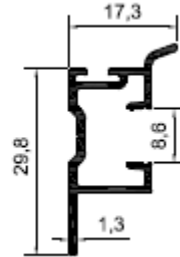
Profil No: N5236 Gramaj : 0,244 kg/mt
