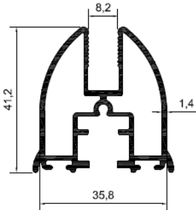
Profil No: 5122 Gramaj : 0,825 kg/mt
